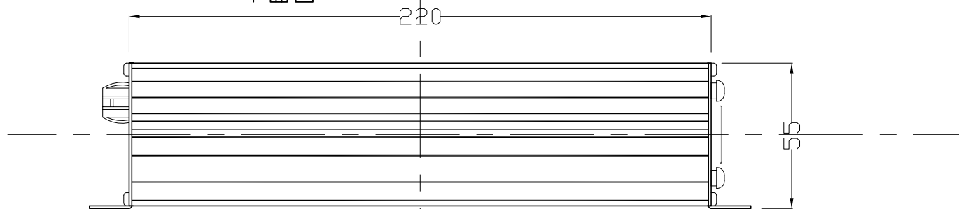
平面図
