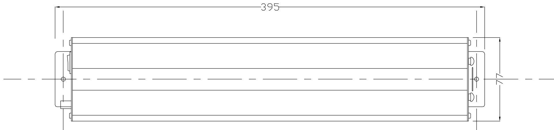
平面図
